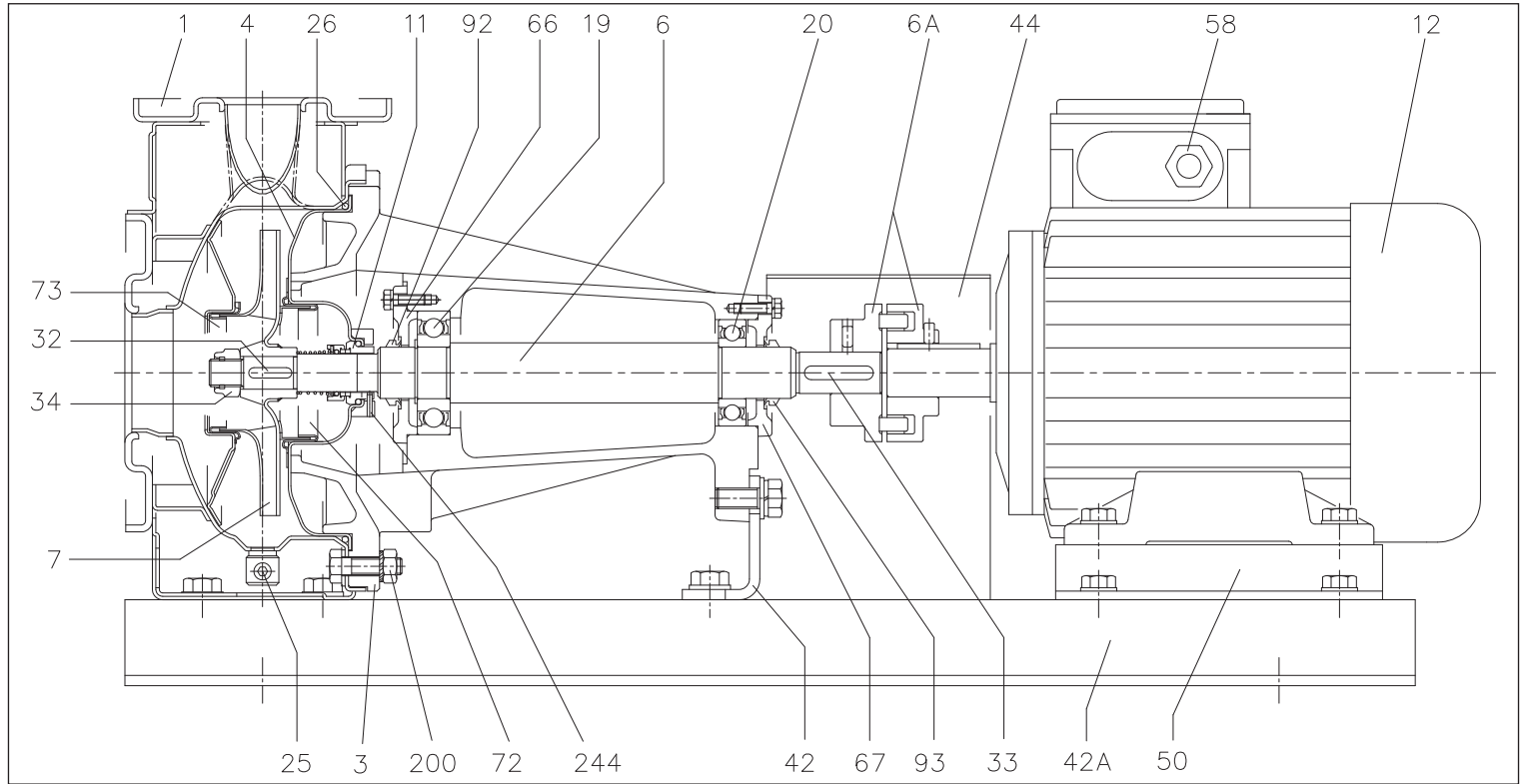
단면도 3(L)P 32, 40, 50, 65-125/160/200
