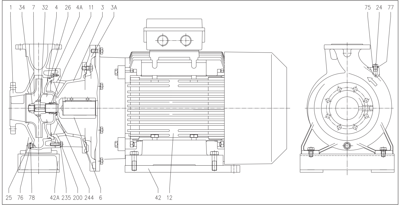
단면도 3LS 65-250,80-200/250
