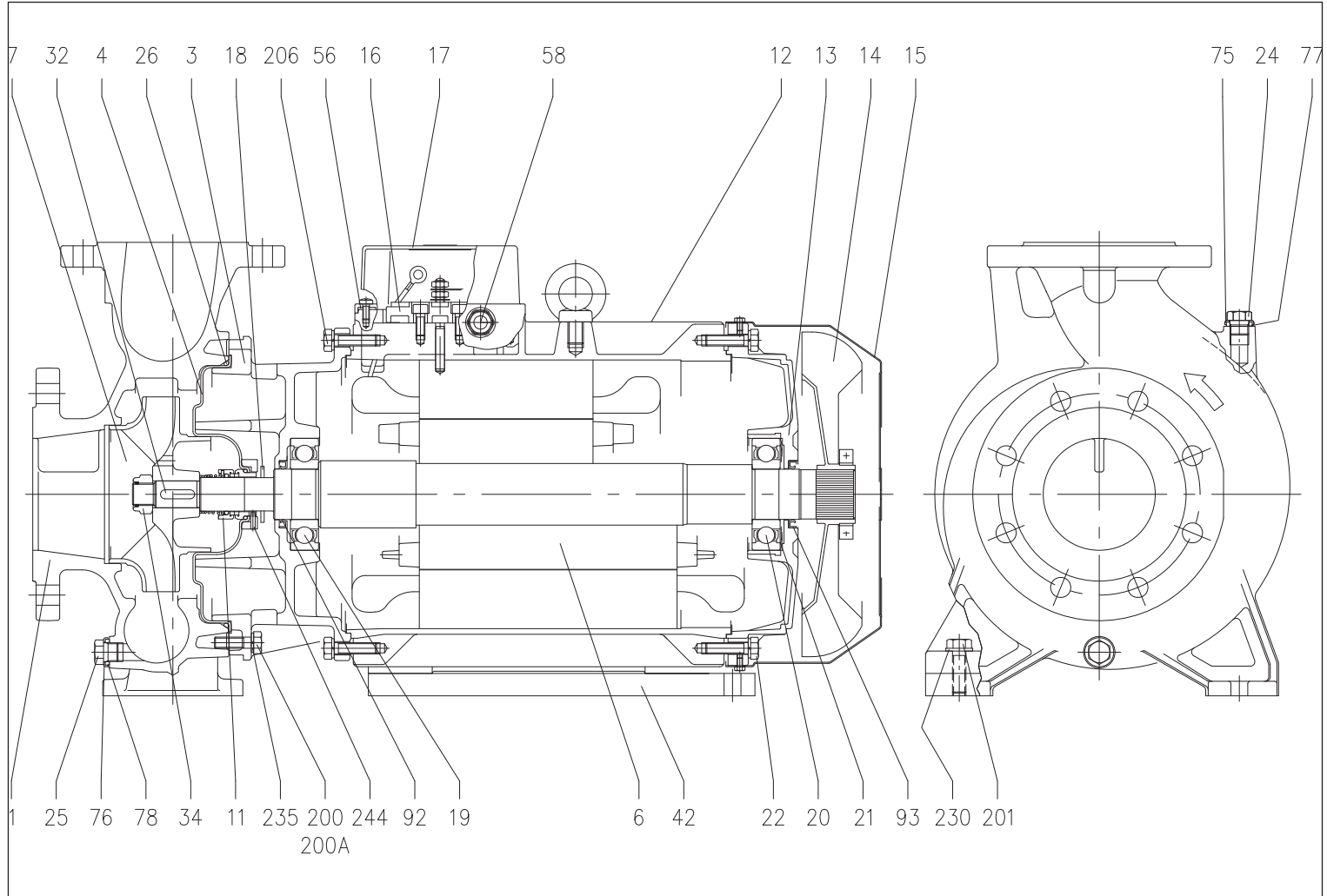
단면도 3LM 80-160
