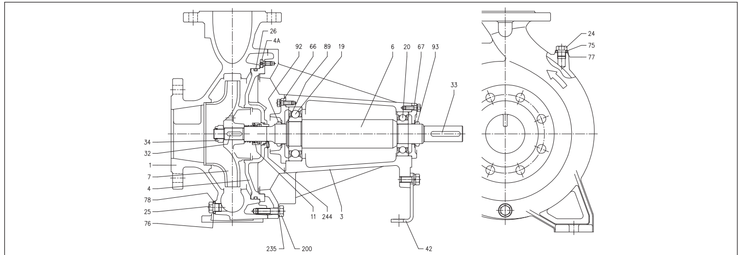
단면도 3LP 65-250, 80-200/250
