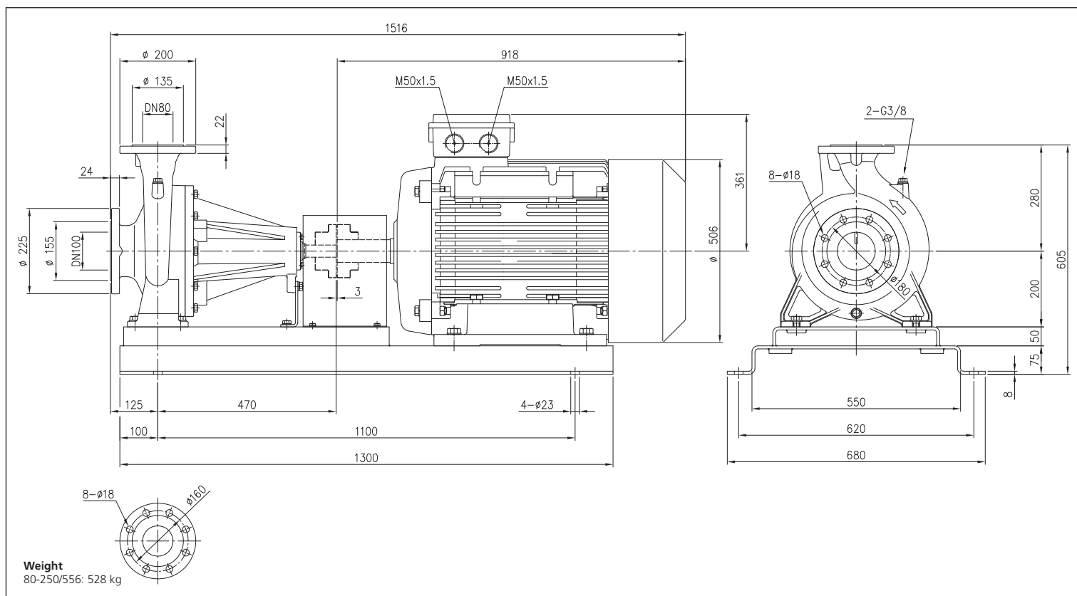
외형도 3LP 80-250/556
