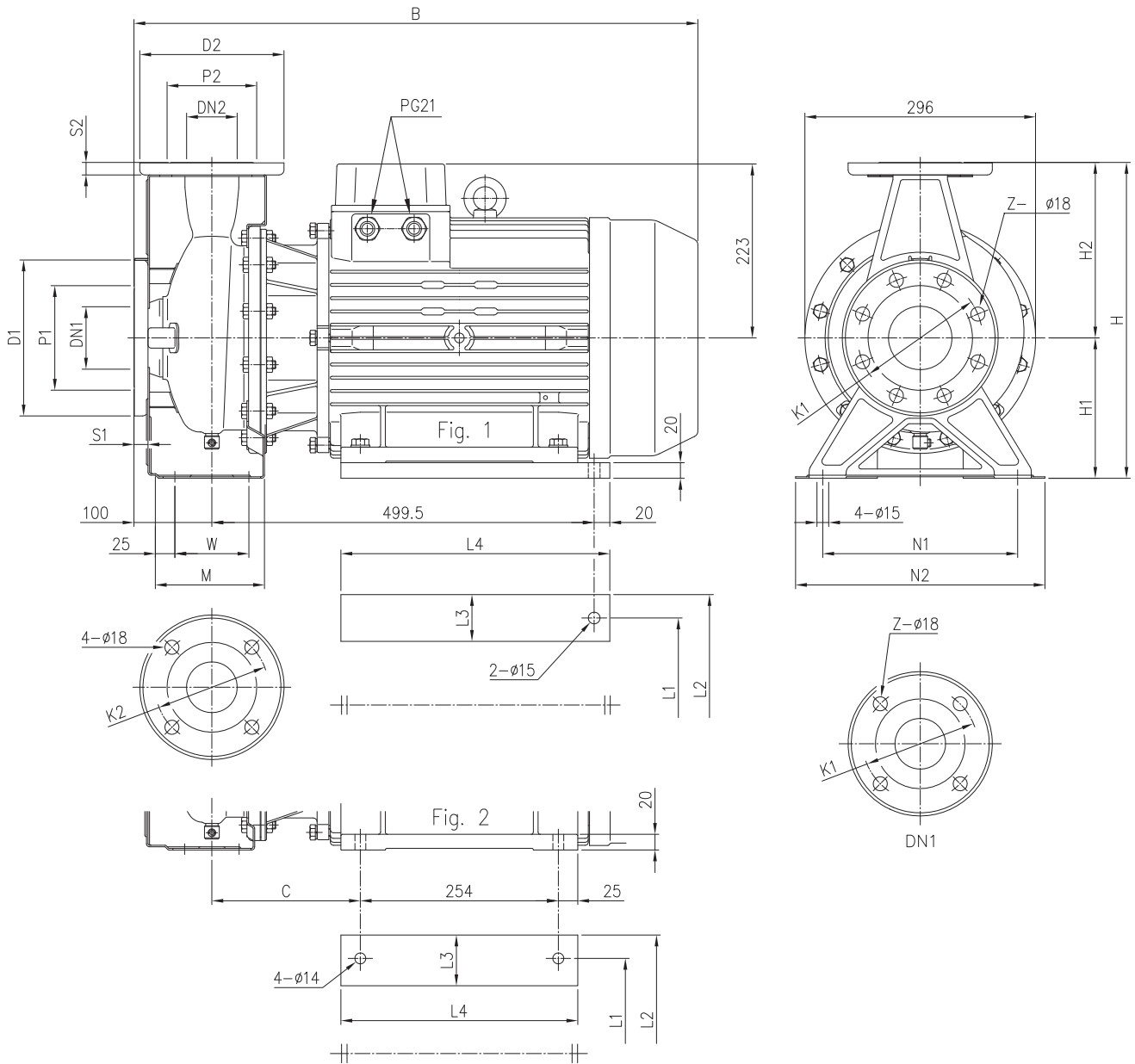
외형도 3(L)M 40-200, 50-160, 65-160/200
