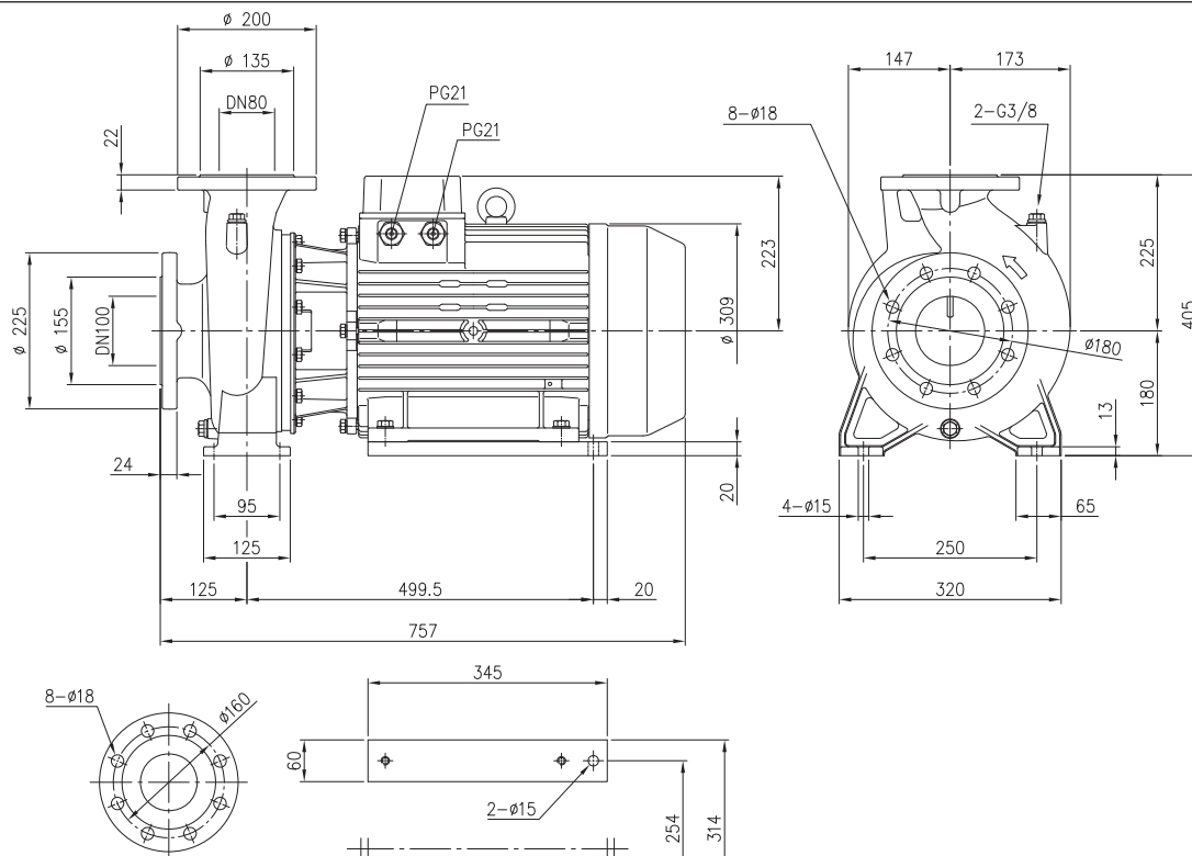
외형도 3LM 80-160/18.56 - 3LM 80-160/226
