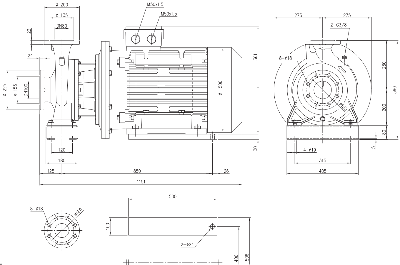
외형도 3LS 80-250/556
