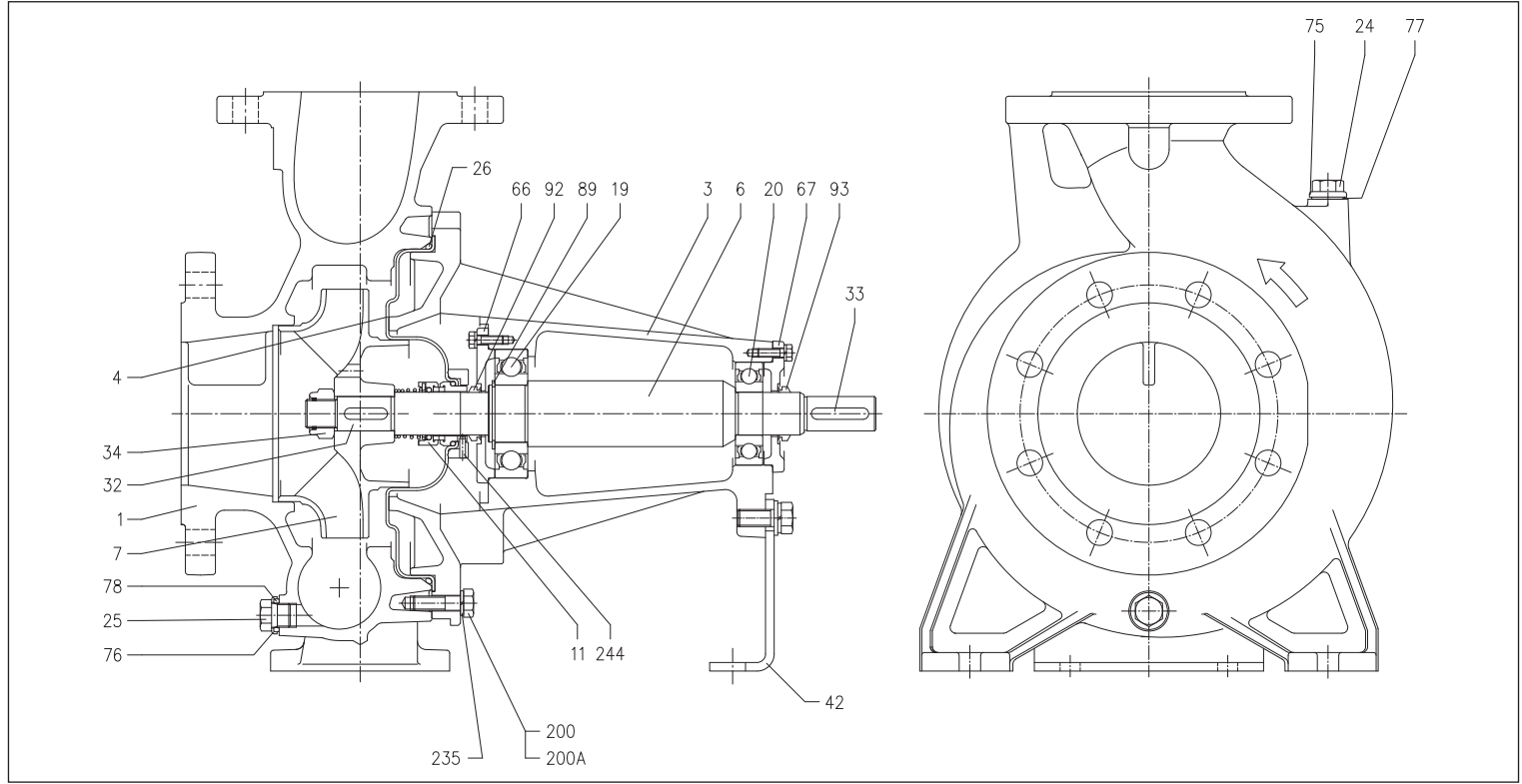
단면도 3LP 80-160
